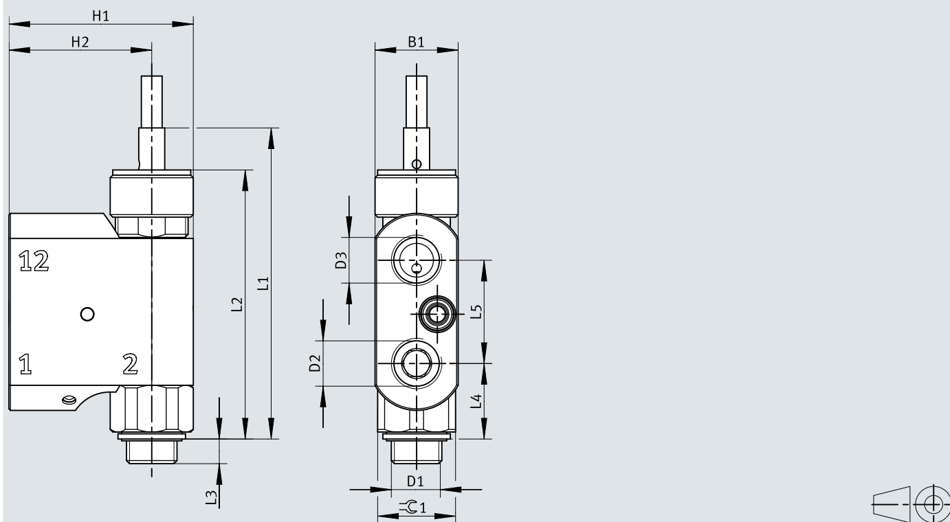
Dimensiones – VBOC-L2-S7-P-M...-G...-E
